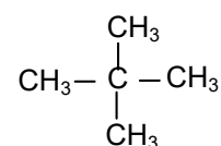
Dimetilpropano
