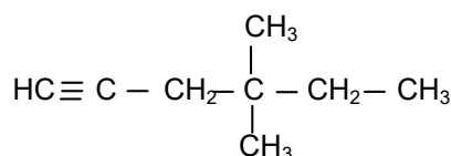
4,4-dimetilhex-1-ino
