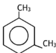
1,3-dimetilbenceno meta-dimetilbenceno m-dimetilbenceno m-xileno
