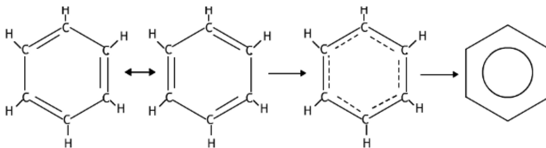
Estructura del anillo bencénico
