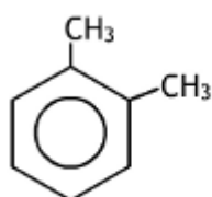
1,2-dimetilbenceno orto-dimetilbenceno o-dimetilbenceno o-xileno
