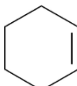
Ciclohexeno
