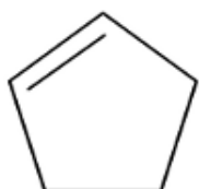
ciclopenteno
