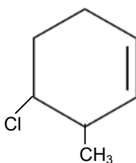
4-cloro-3-metilciclohexeno
