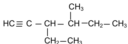
3-etil-4-metilhex-1-ino
