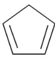
ciclopenta-1,3-dieno
